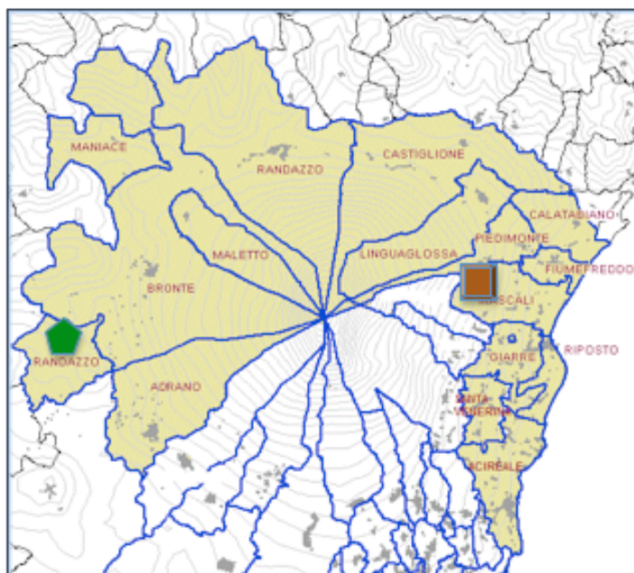
Figura 6 - Mappatura localizzazione impianti di trattamento
